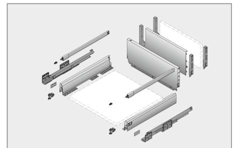
ArciTech flexible Sets, weiß Höhen 94, 126, 186 und 218 mm Zubehör
