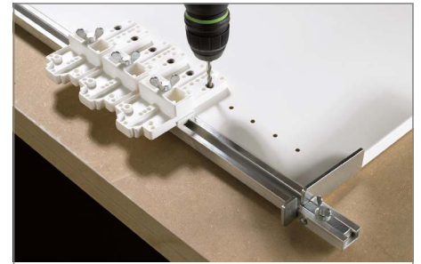
Exakta Bohrlehre
