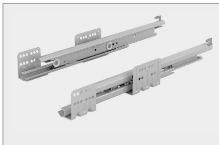
Actro mit Silent System Auszugsführungen und Öffnungssystem Push to open Silent für Korpusseitendicke 18 / 19 mm
