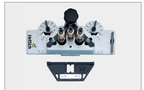
Bohrlehre DrillJig, Scharniere
